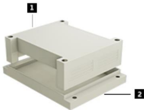
爆炸图
