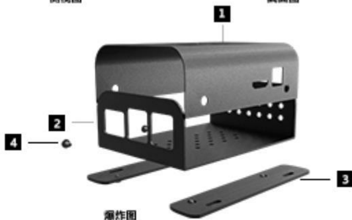
爆炸图
