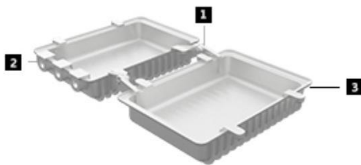
爆炸图
